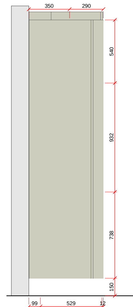
VISTA A - LATERAL - ESC. 1:20
