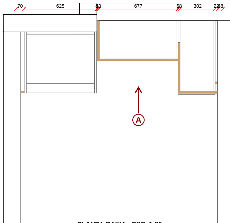
PLANTA BAIXA - ESC. 1:20
