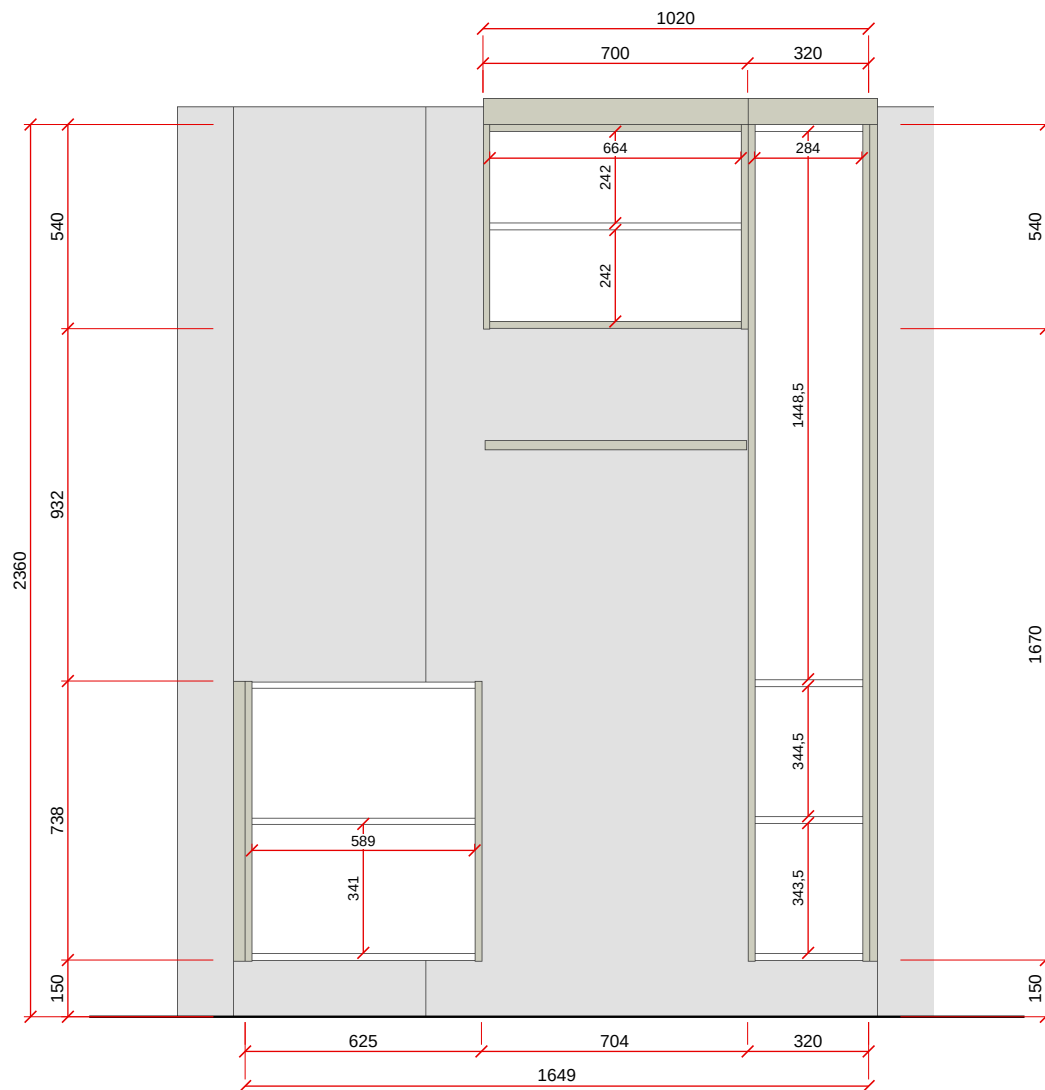
VISTA A - ESC. 1:20
